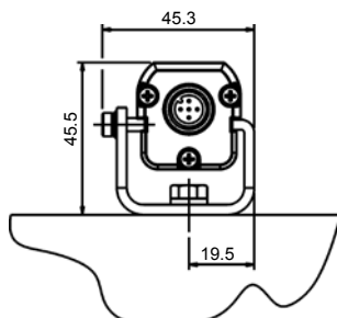
Serie SF2: applicazione con staffa standard di fissaggio. La staffa di fissaggio standard è compatibile con la staffa standard SE, supporto anti-vibrazioni ST-K*AV.
