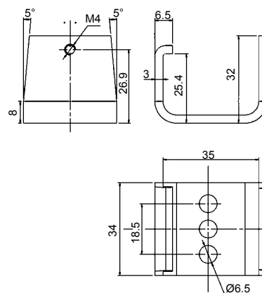
Serie SF2: staffa standard di fissaggio.
