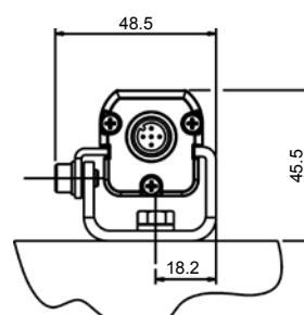
Serie SF2: applicazione con staffa anti-graffio ST-KSF2.
