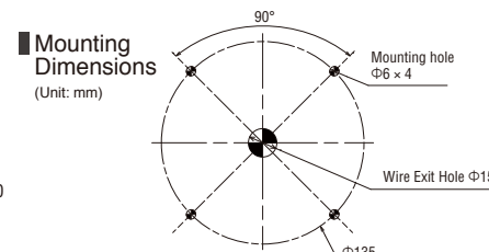
Circular Bracket (For \Phi 100\text{mm} ) SZW-101
