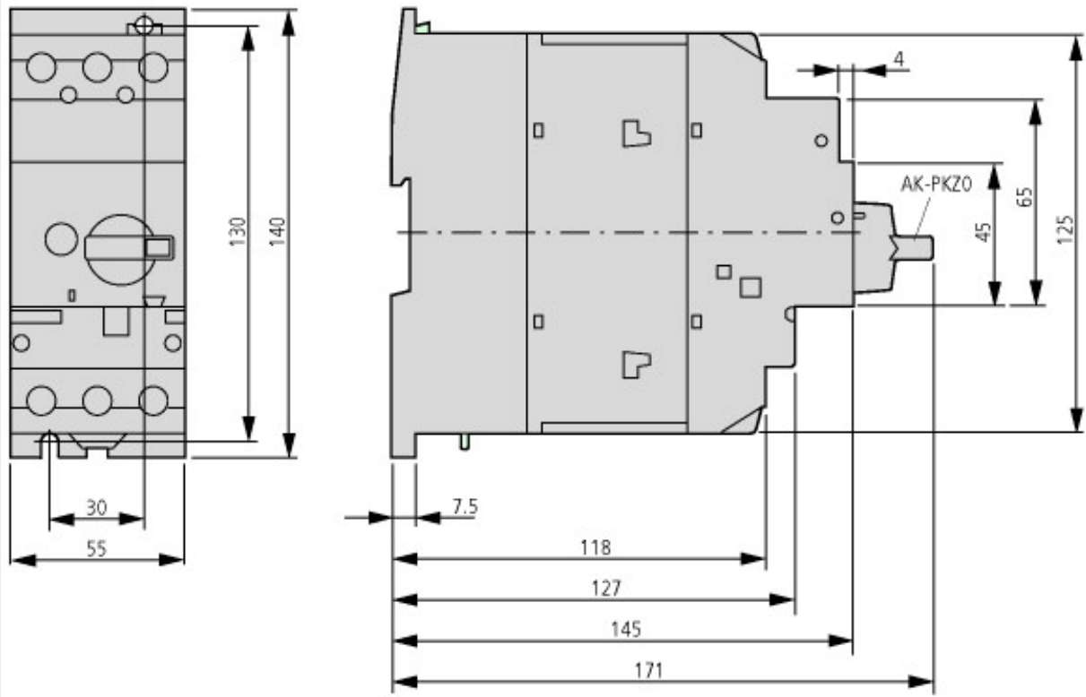
PKZM4-... +AK-PKZ0
