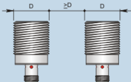
Montaggio affiancato
