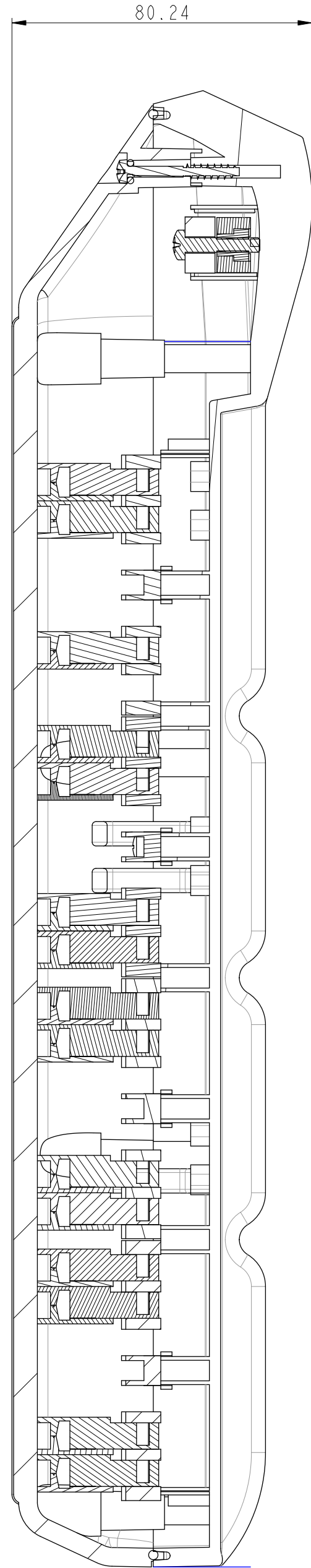
SEZIONE XSEC0002-XSEC0002
