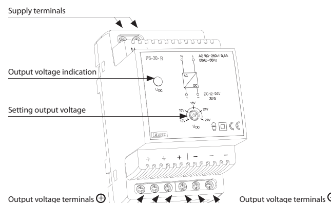
PS-30-R
