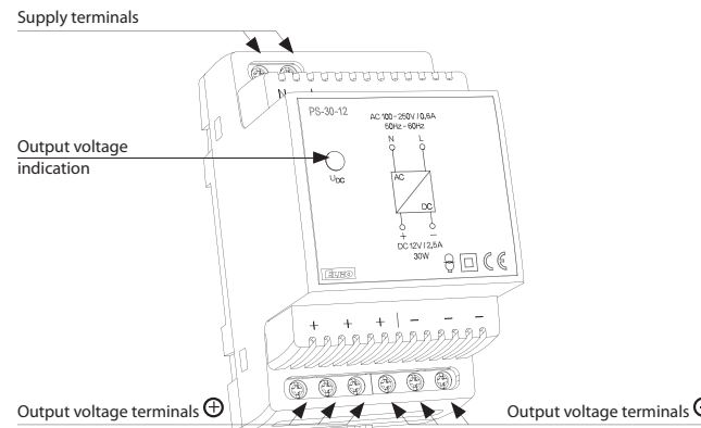
PS-30-12
