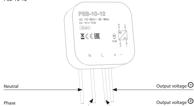
PSB-10-12
